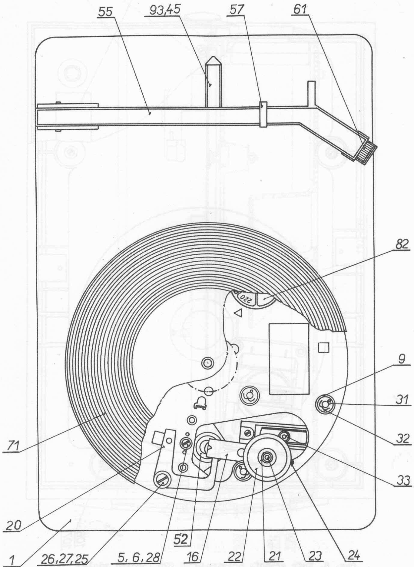
Obr. 7. Pohled na chassis shora
