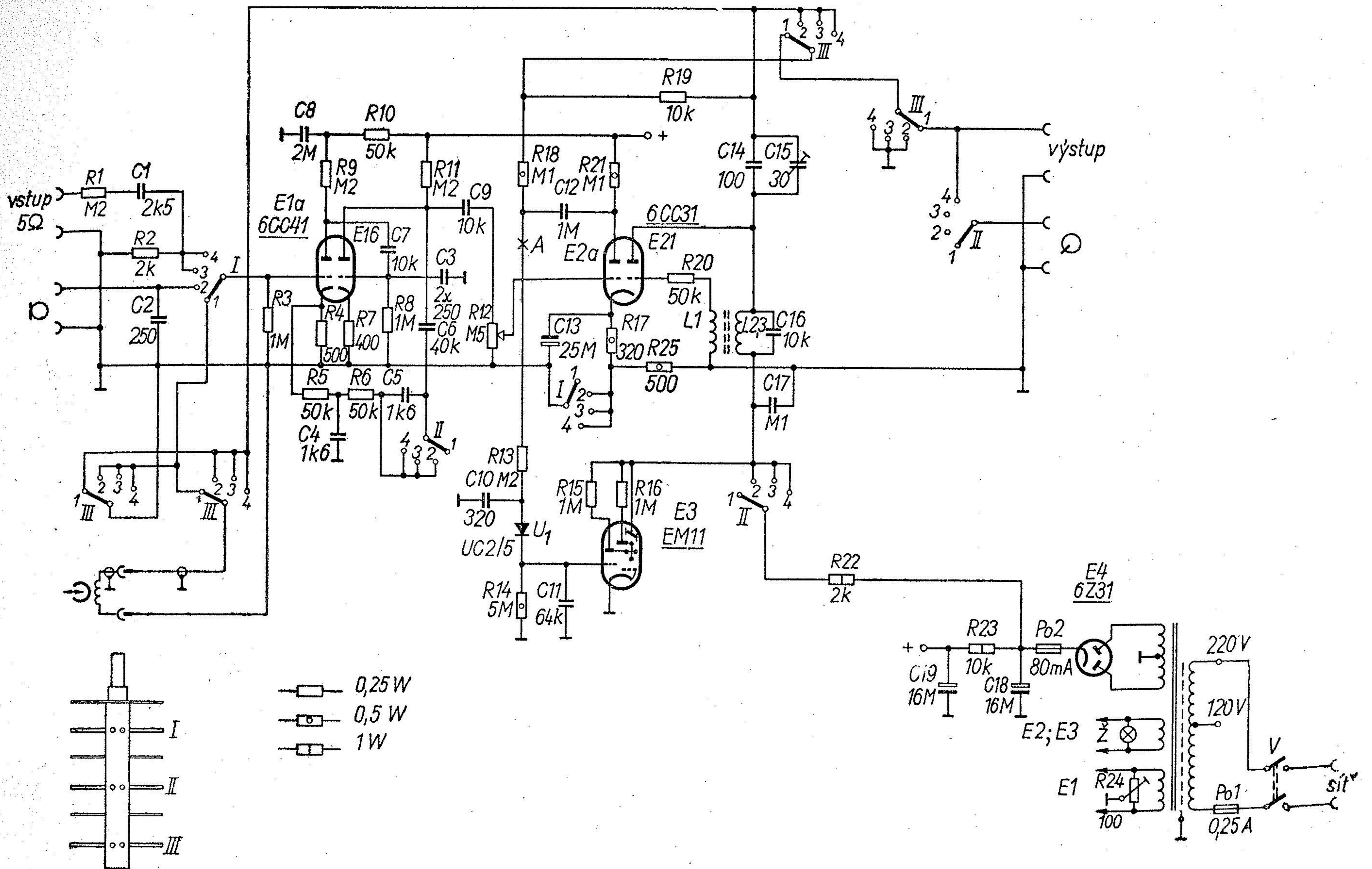
Obr. 11. Zapojení adaptoru TESLA 2 AN 380 00 (elektronky E16 a E21 mají být označeny E1b a E2b)
