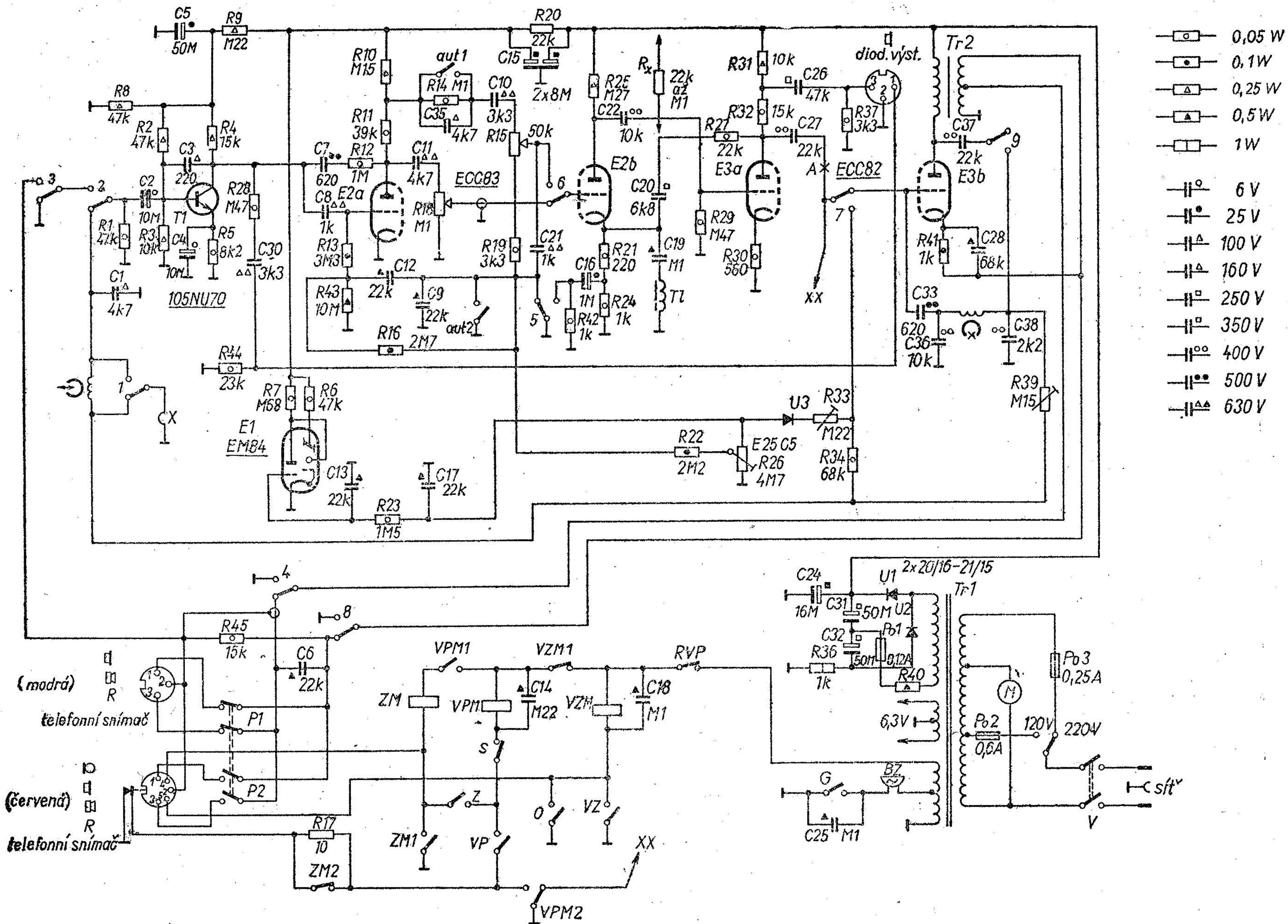
Obr. 14. Zapojení diktafonu TESLA AKTIV ANP 302
