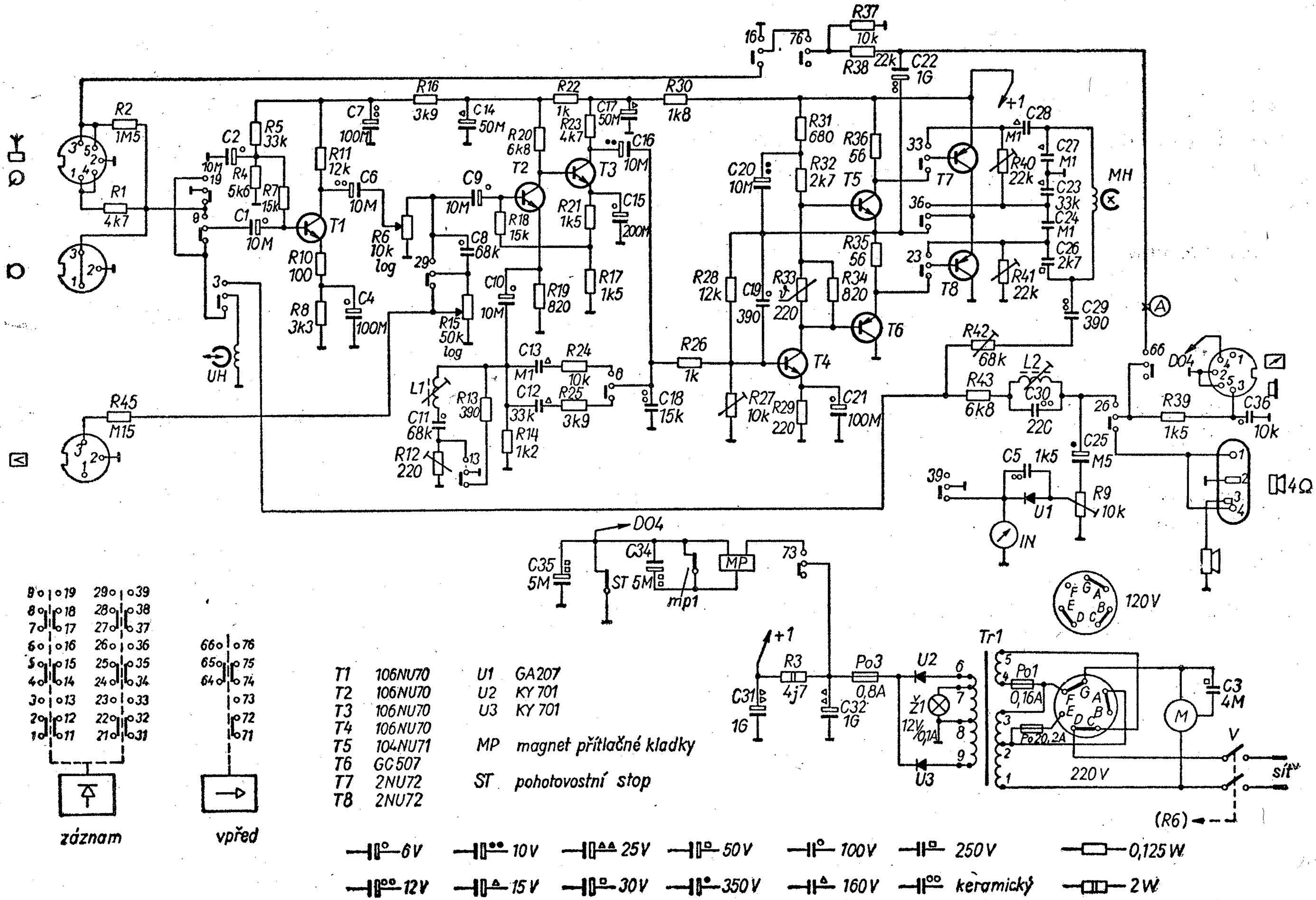
Obr. 106. Zapojení magnetofonů TESLA B 41, B 44
