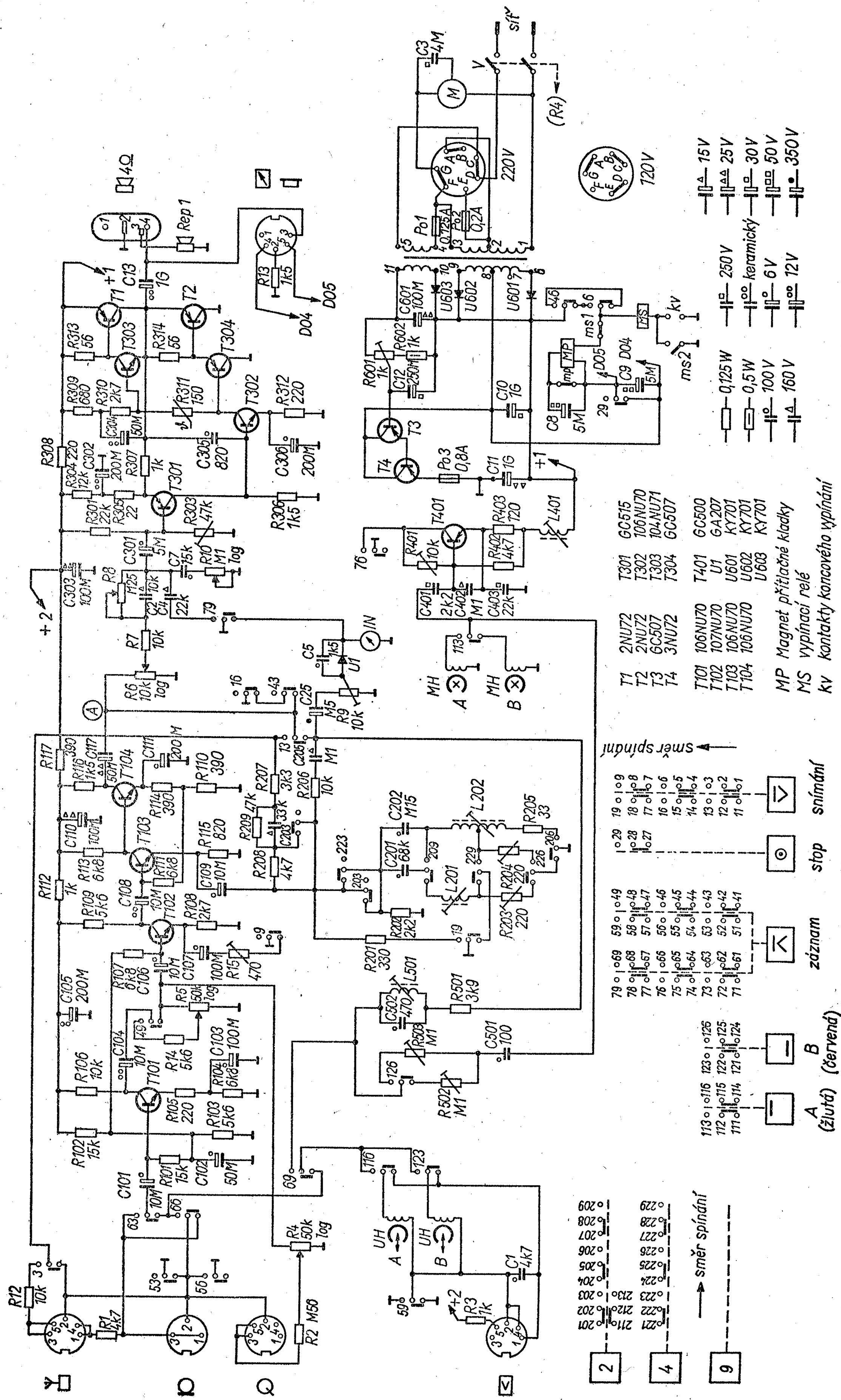
Obr. 104. Zapojení magnetofonu TESLA 444 LUX ANP 240
