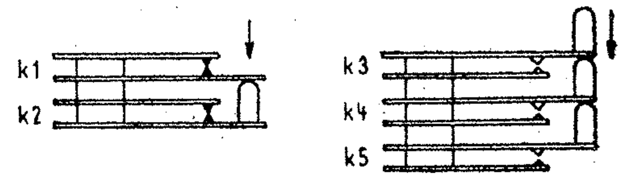
propojovací svorkovnice
