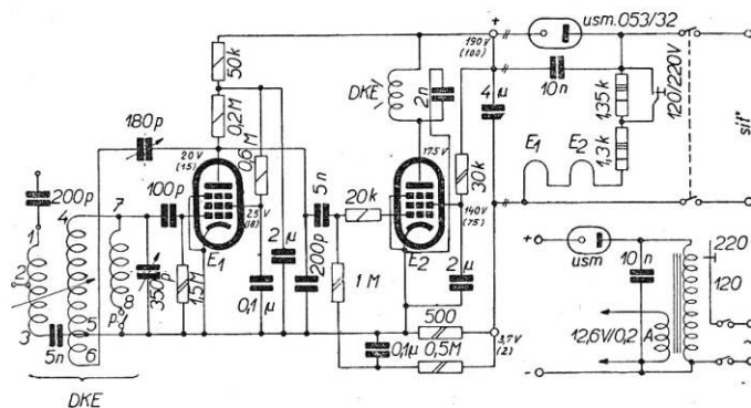
Obr. 2: Schéma stavebnice DKE z čas. Radioamatér
