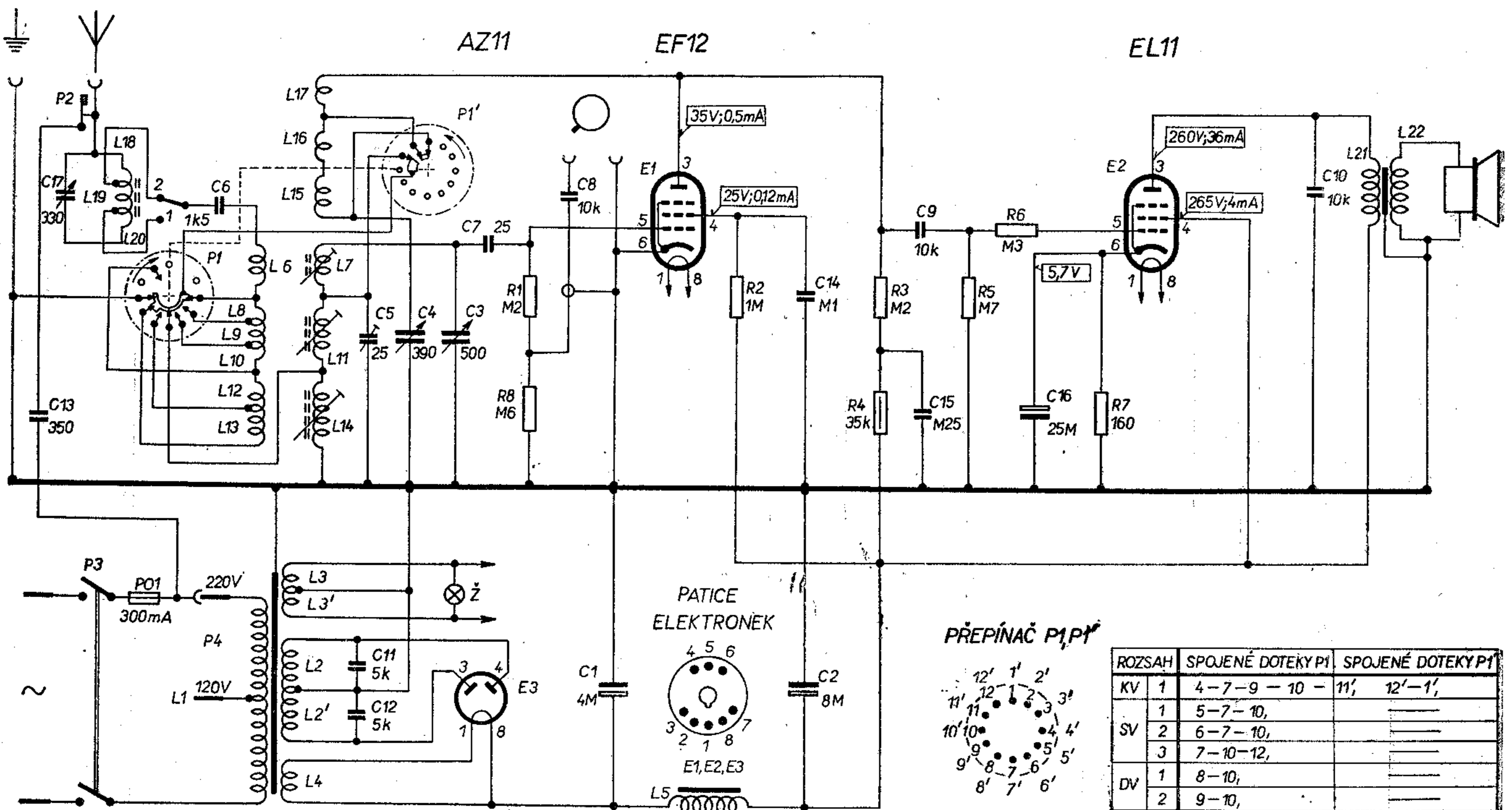
Zapojení přijímače T 613
